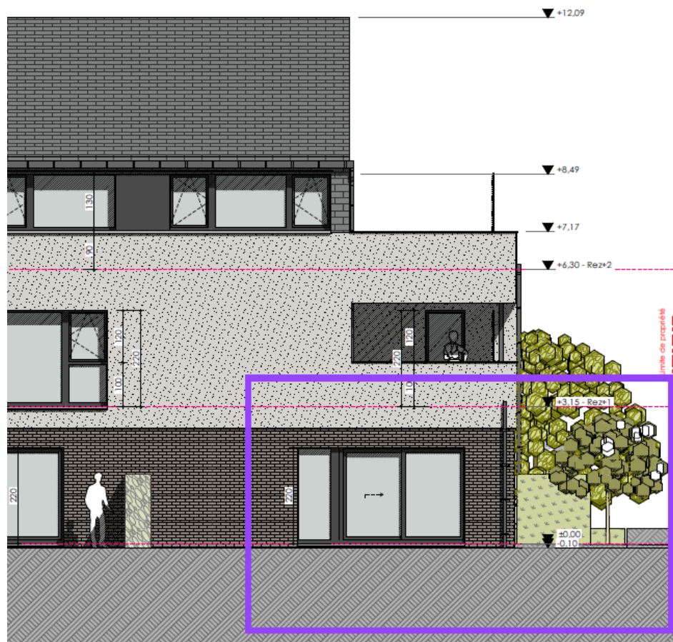
Façade arrière
